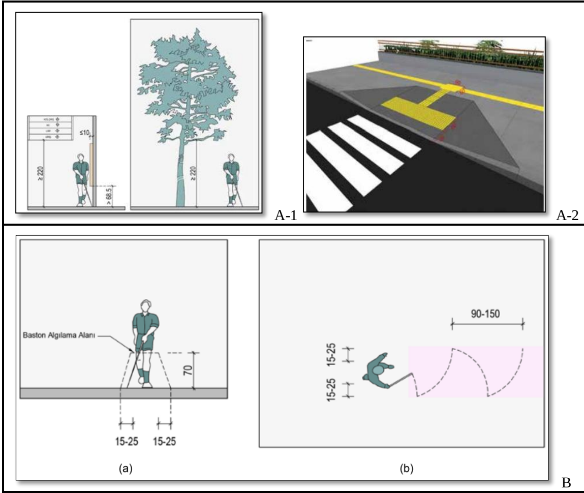
Şekil 4. A1- Dikeyde engelsiz alan ölçüleri. A-2 Üç yöne eğimli rampalı, hissedilebilir yüzeyli yaya yolu (iz yolu). B- Beyaz Baston kullanımı için gerekli mesafe (Çağlayan, 2020).
